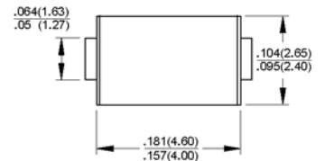
DO-214AC (SMA)
