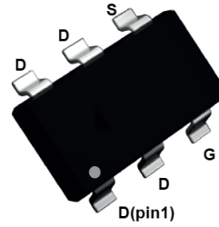
SOT-23-6L
